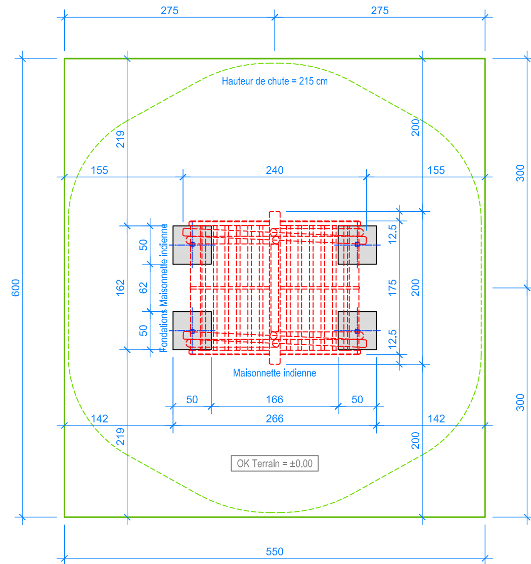
PLAN 1:50
