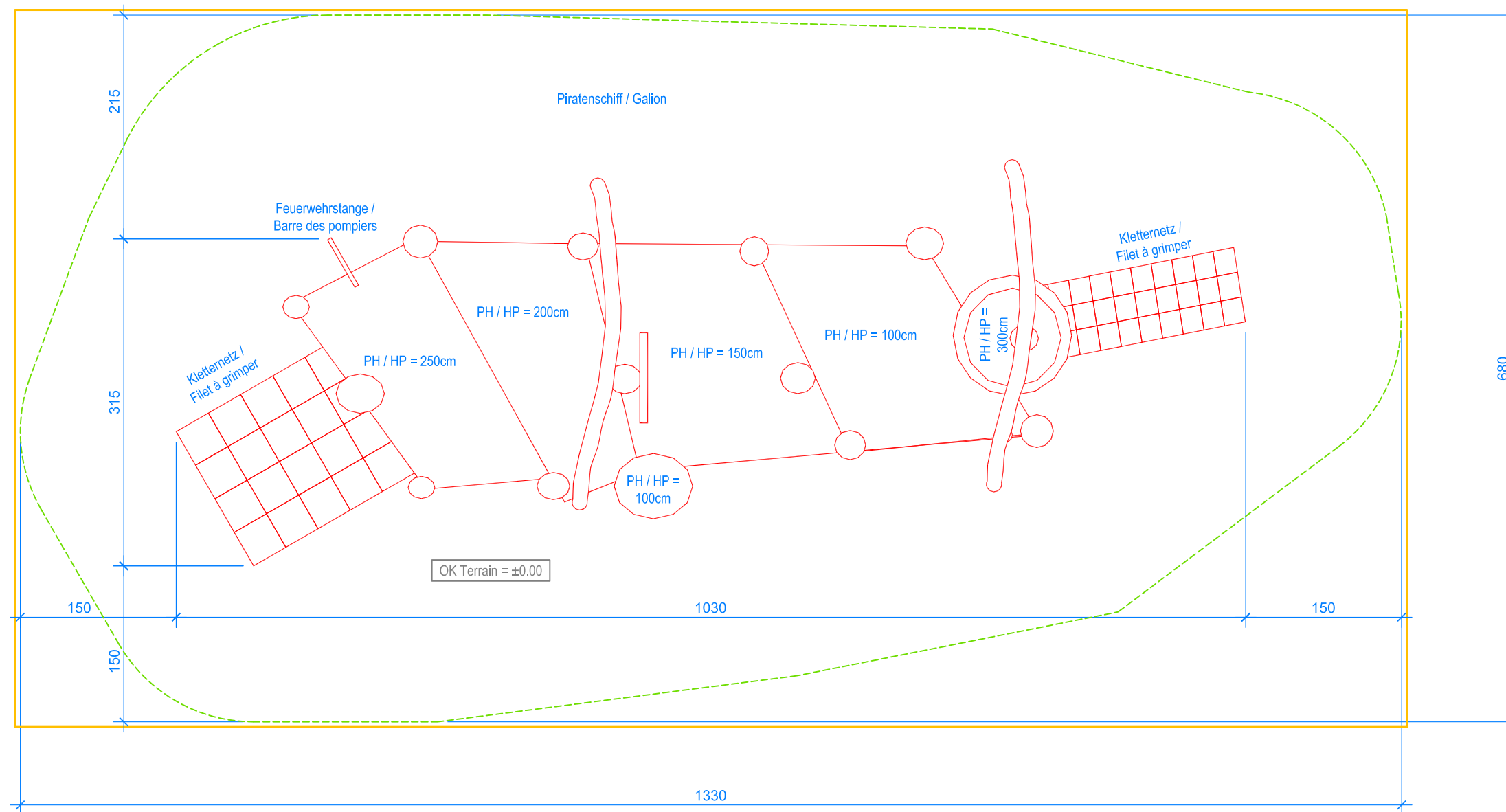
GRUNDRISS / PLAN 1:50
