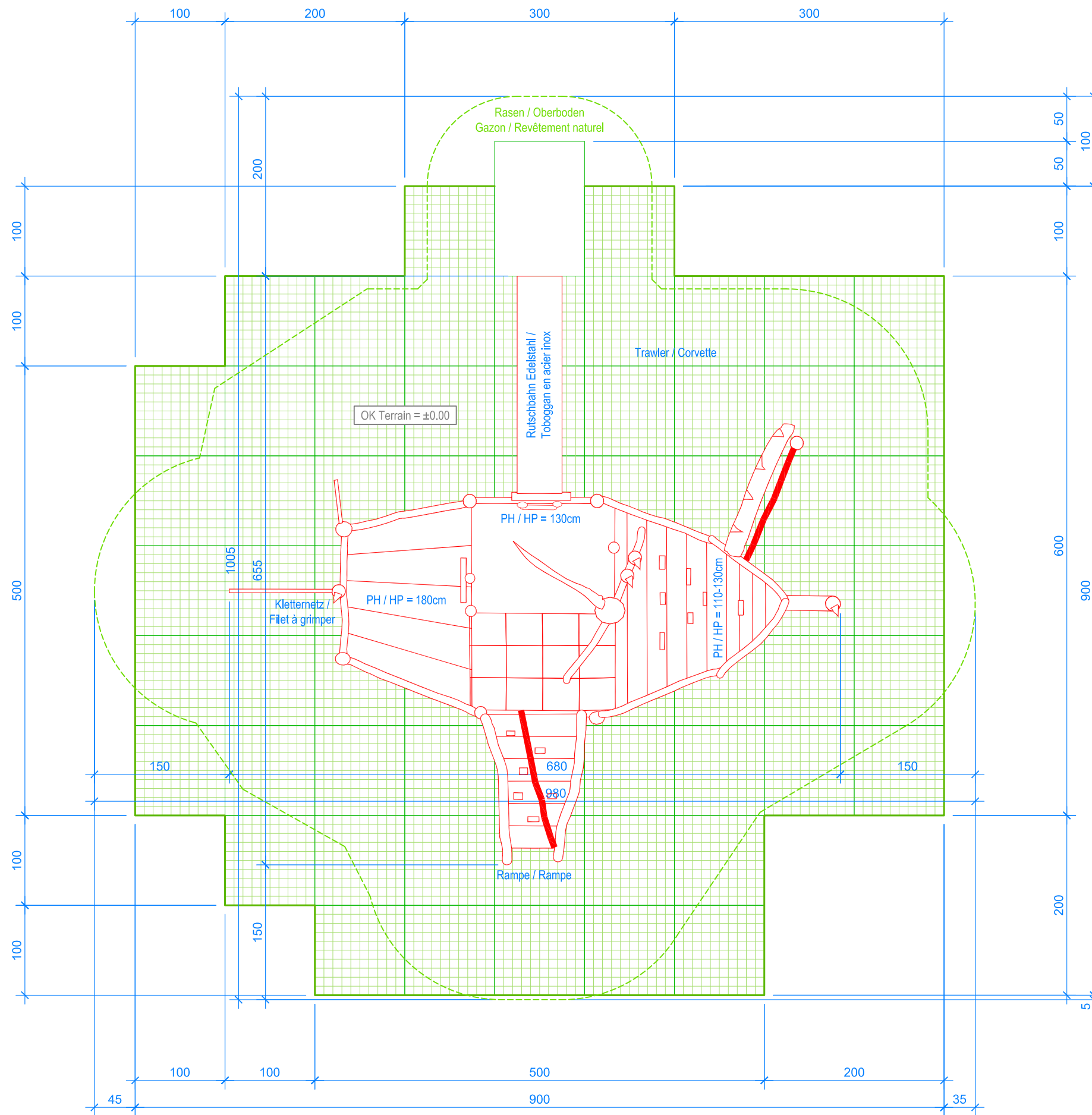
GRUNDRISS / PLAN 1:50
