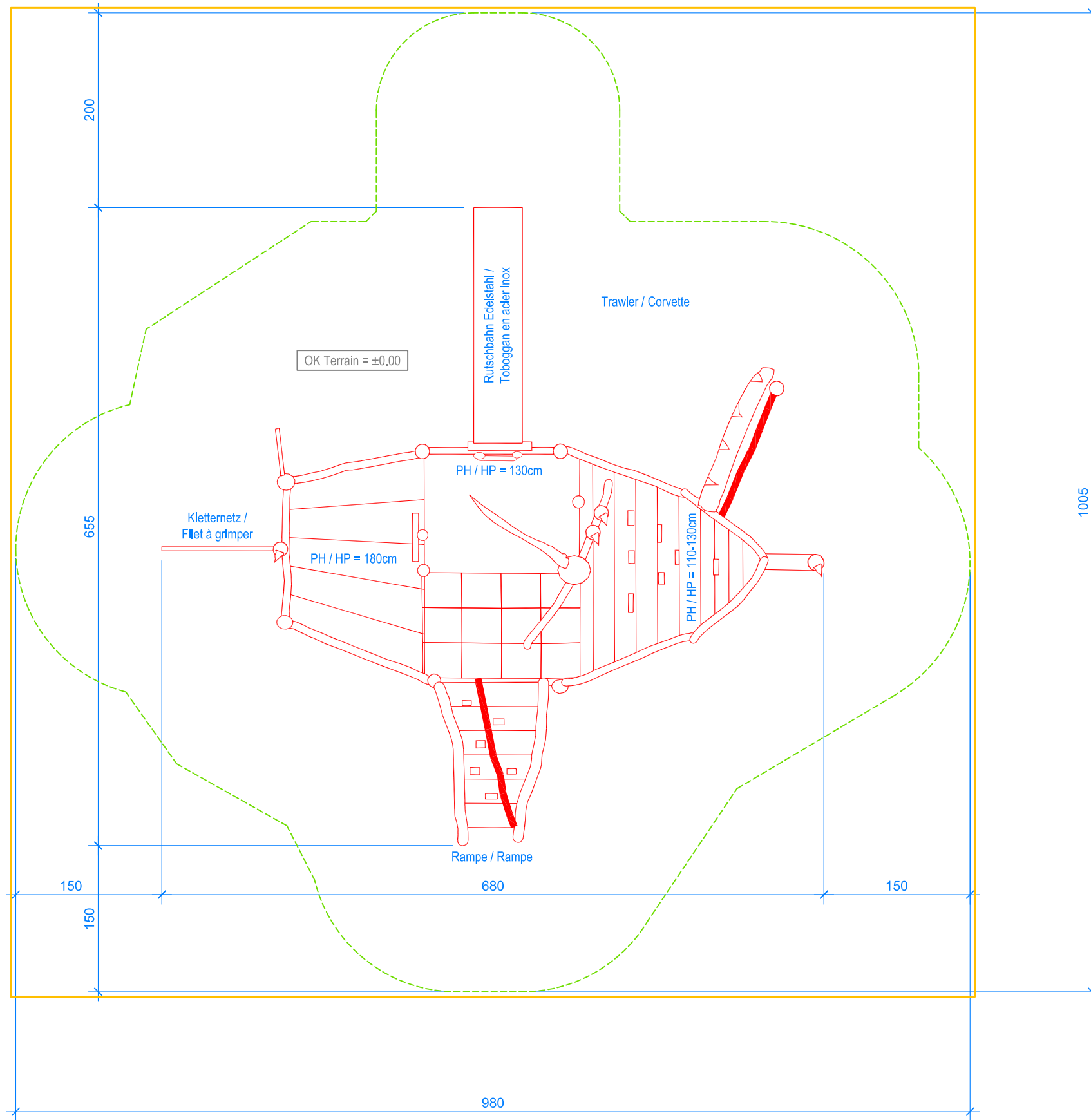
GRUNDRISS / PLAN 1:50
