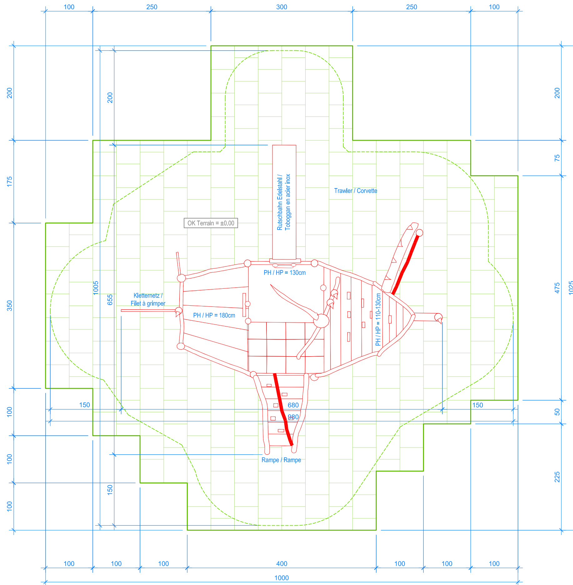
GRUNDRISS / PLAN 1:50
