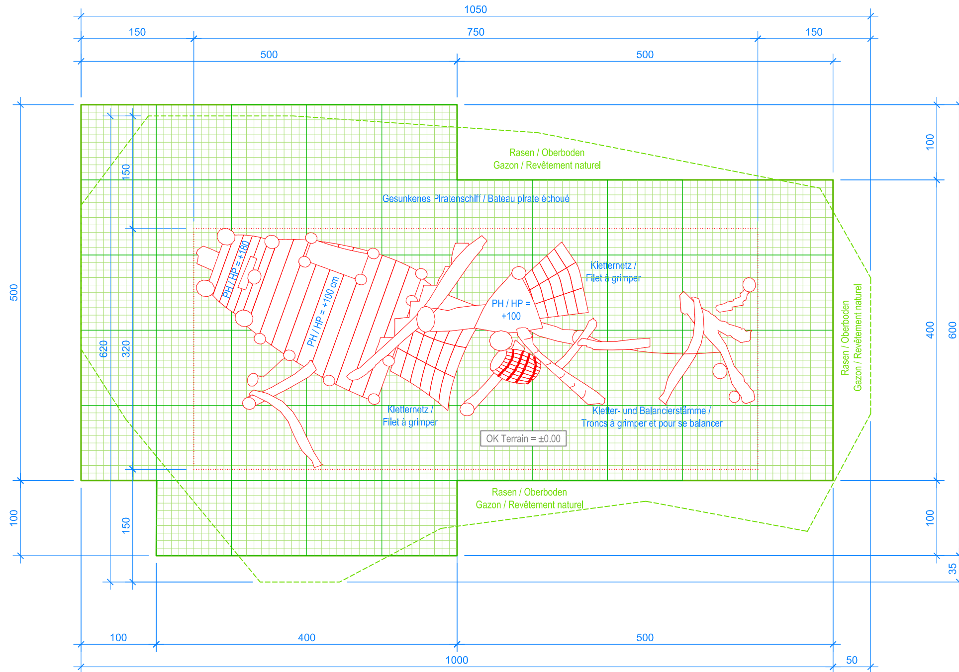
GRUNDRISS / PLAN 1:50
