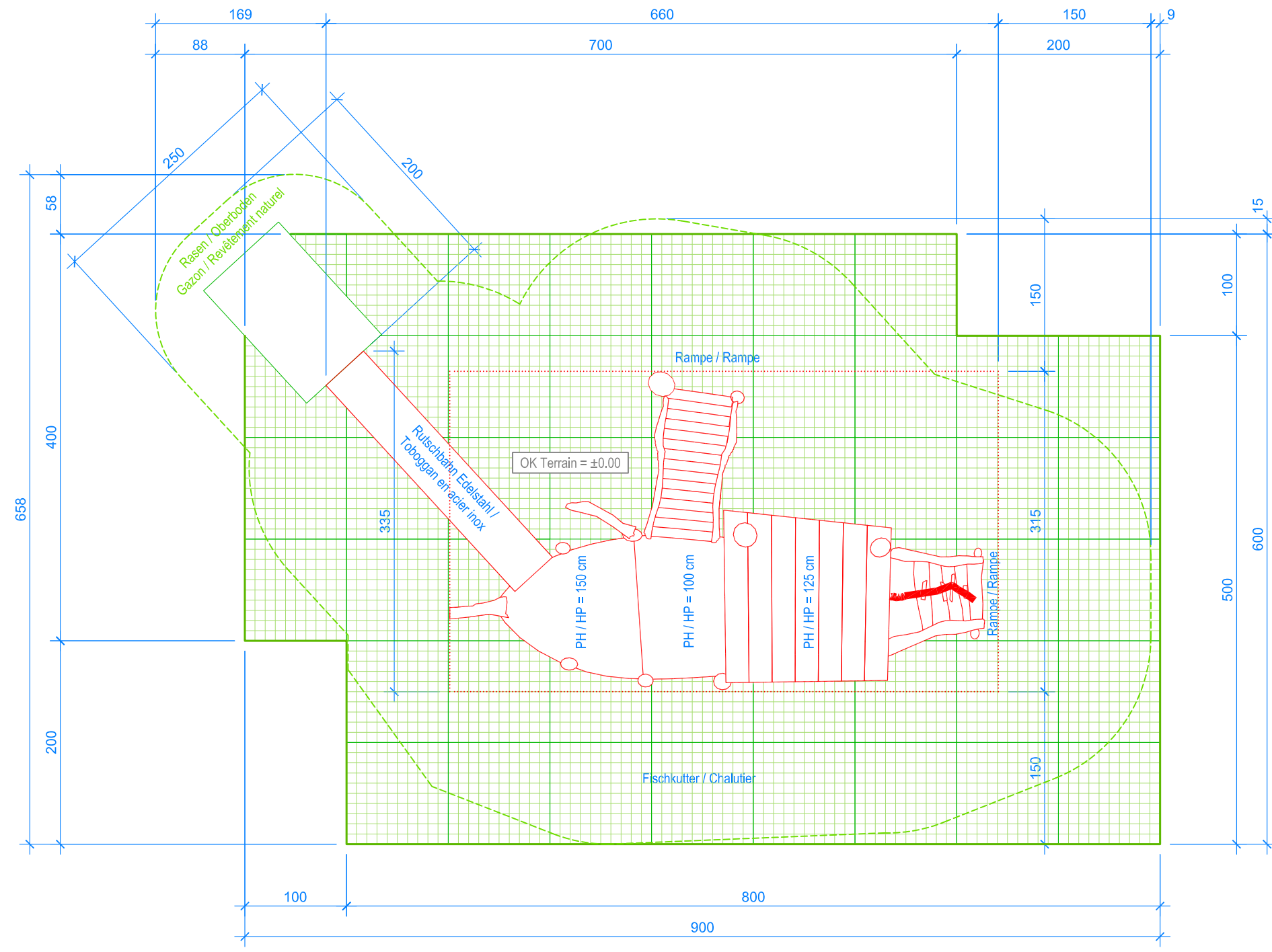
GRUNDRISS / PLAN 1:50
