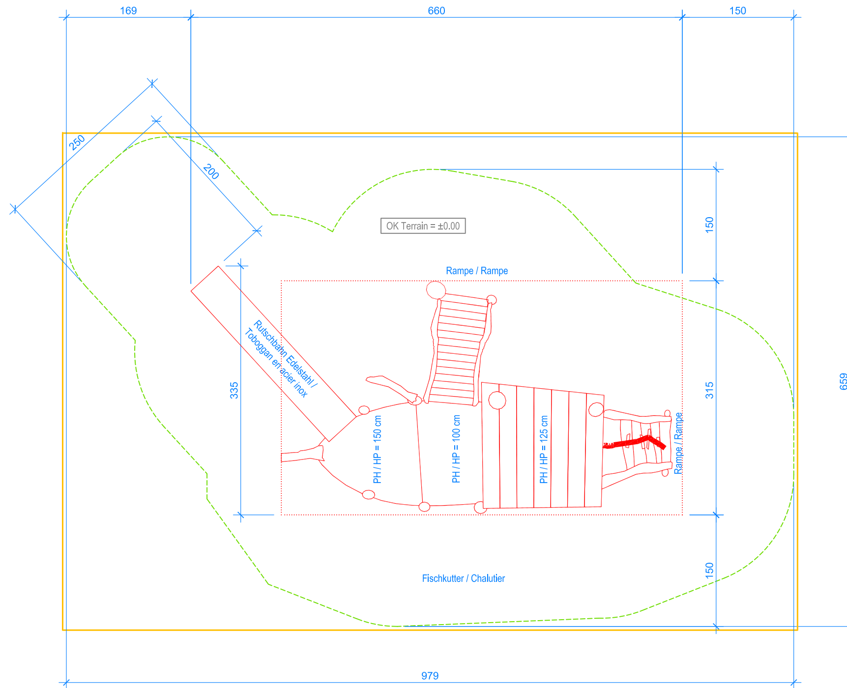
GRUNDRISS / PLAN 1:50
