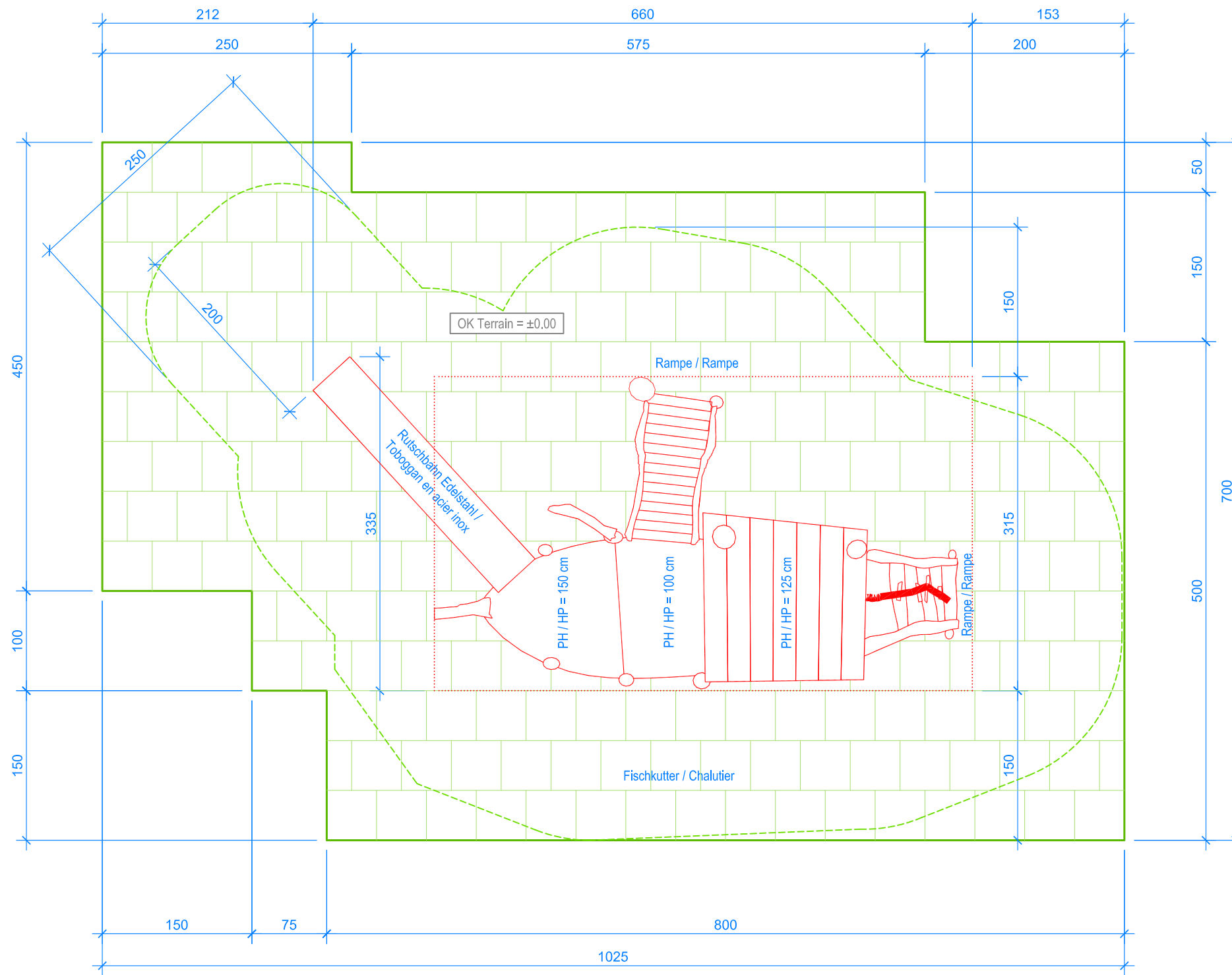
GRUNDRISS / PLAN 1:50
