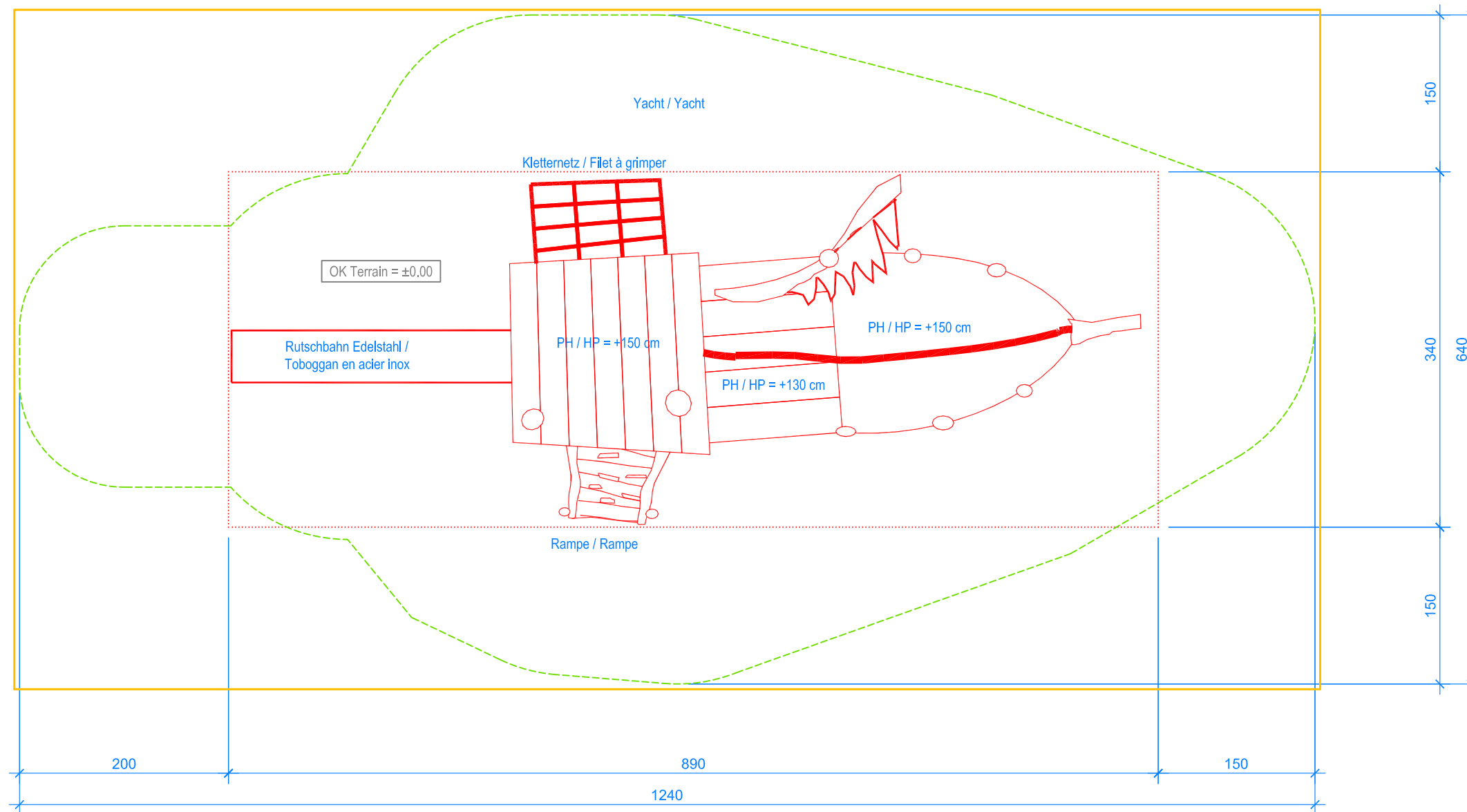
GRUNDRISS / PLAN 1:50
