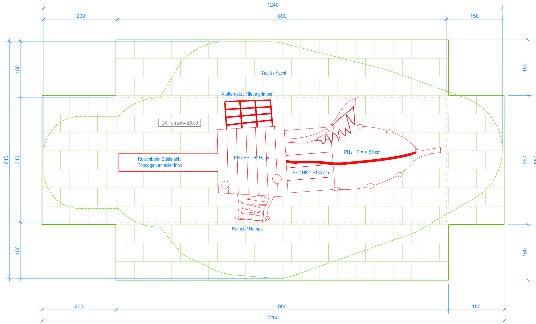
GRUNDRISS / PLAN 1:50
