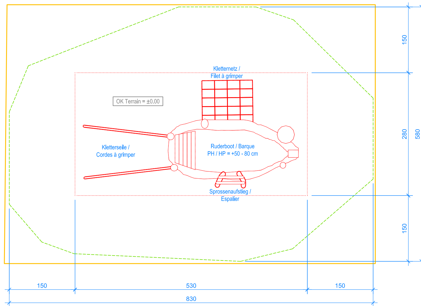
GRUNDRISS / PLAN 1:50
