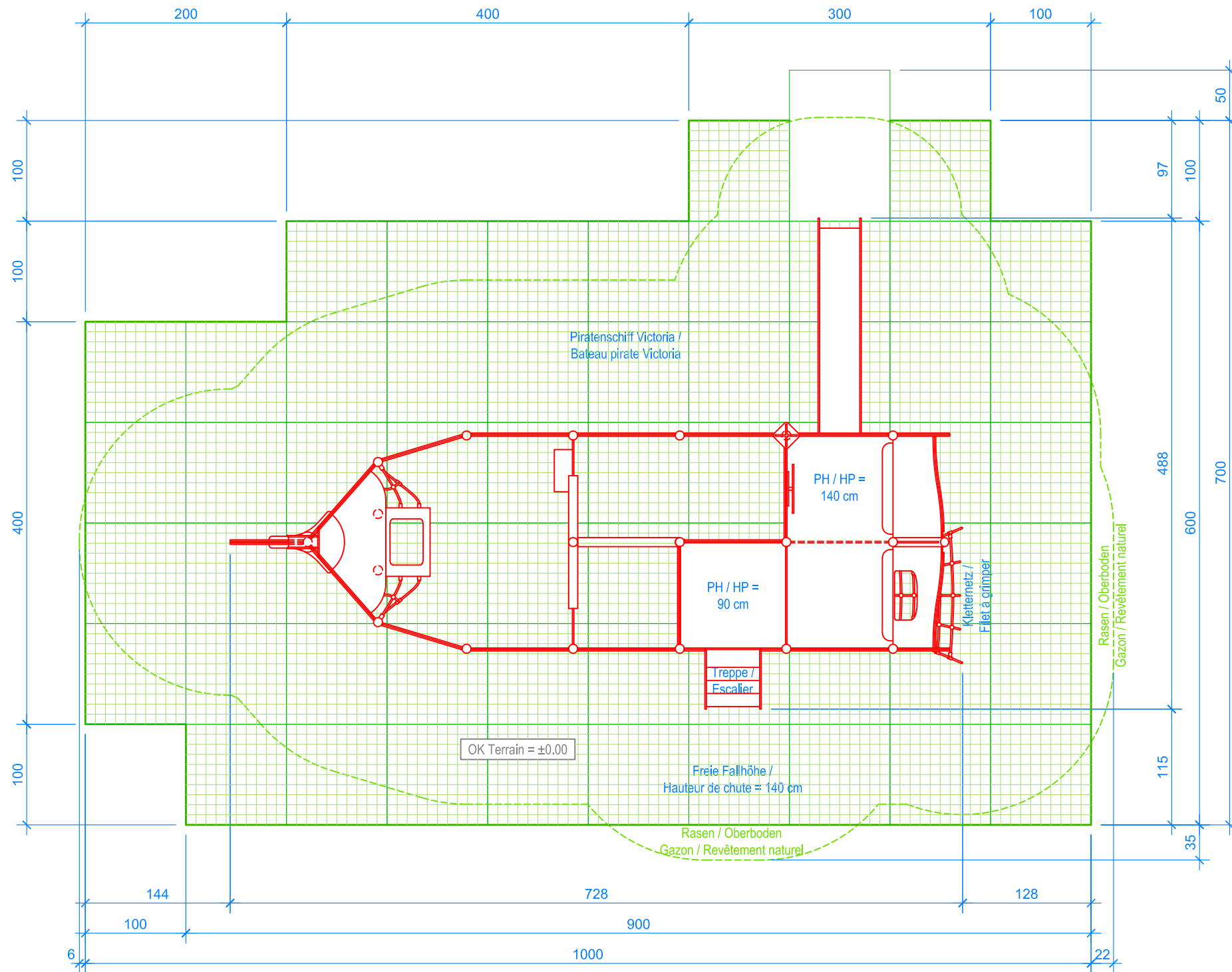
GRUNDRISS / PLAN 1:50
