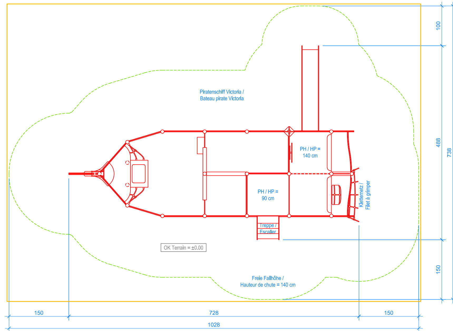
GRUNDRISS / PLAN 1:50
