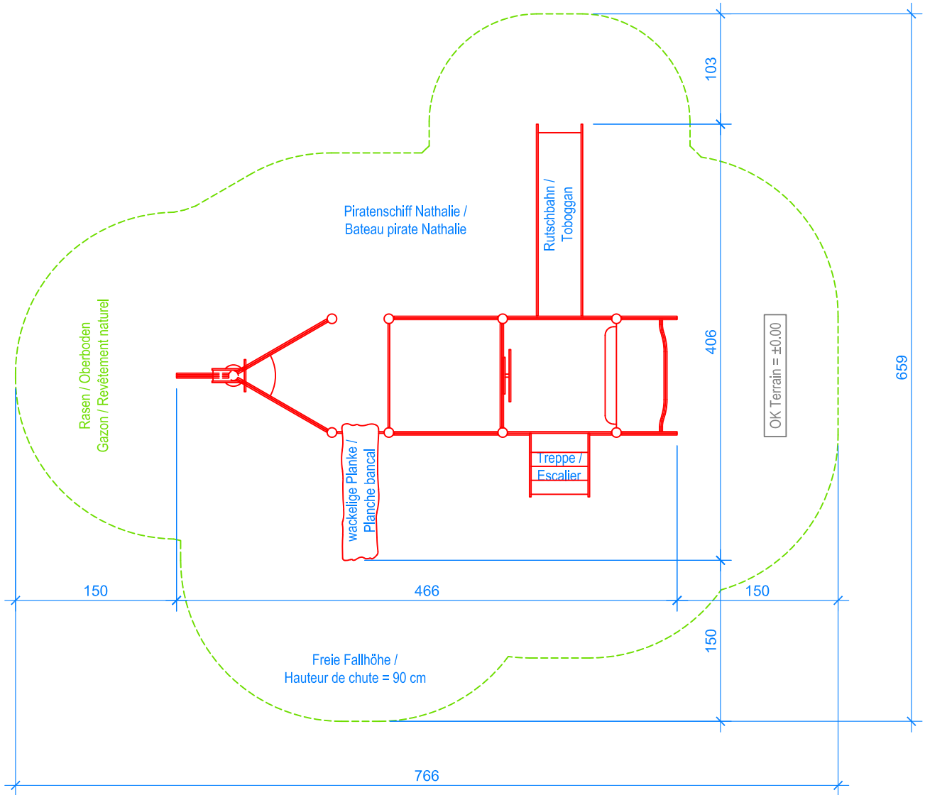
GRUNDRISS / PLAN 1:50
