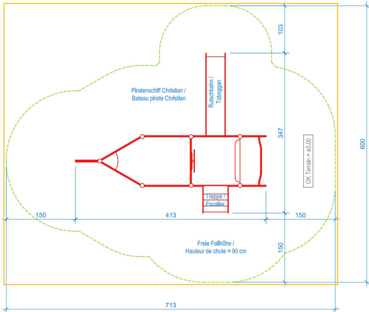
GRUNDRISS / PLAN 1:50
