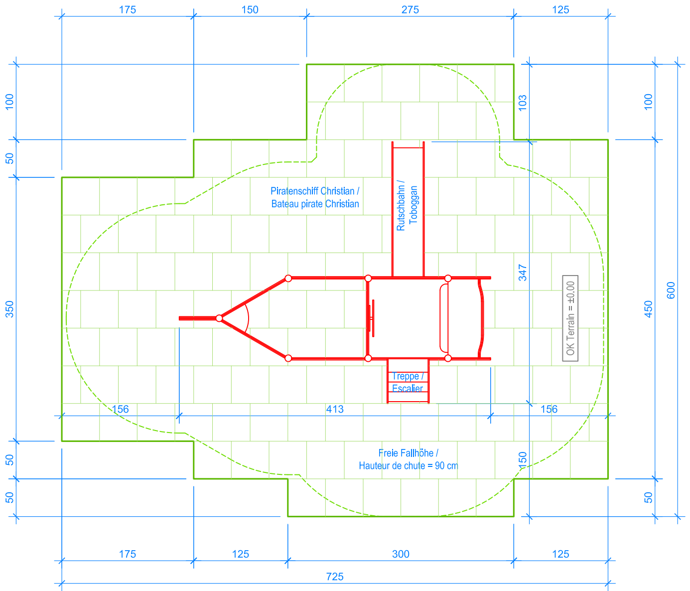
GRUNDRISS / PLAN 1:50
