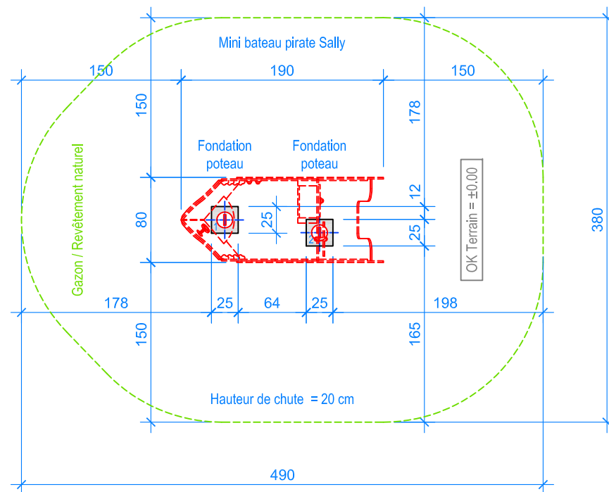
PLAN 1:50
