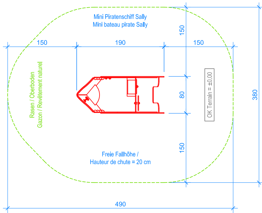
GRUNDRISS / PLAN 1:50
