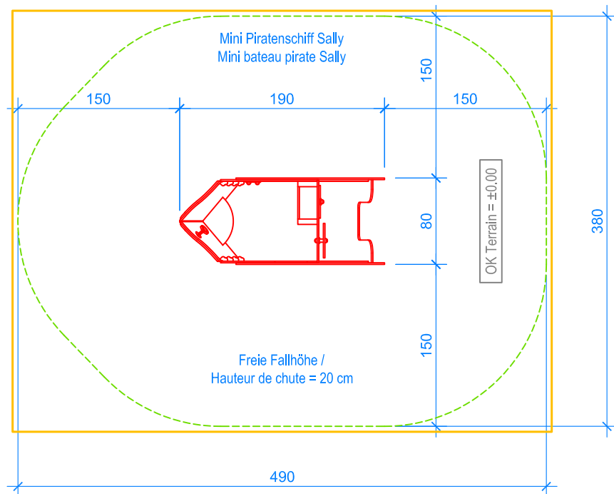
GRUNDRISS / PLAN 1:50
