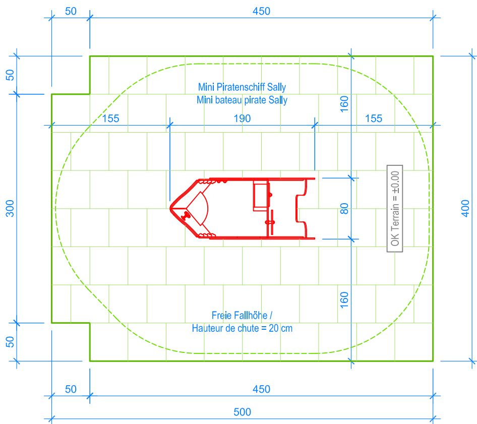
GRUNDRISS / PLAN 1:50
