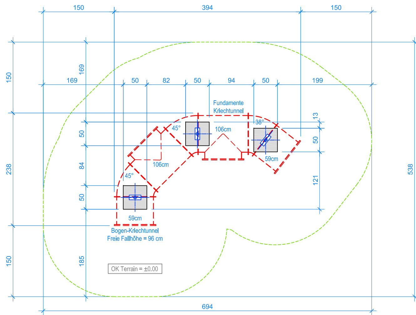
GRUNDRISS 1:50
