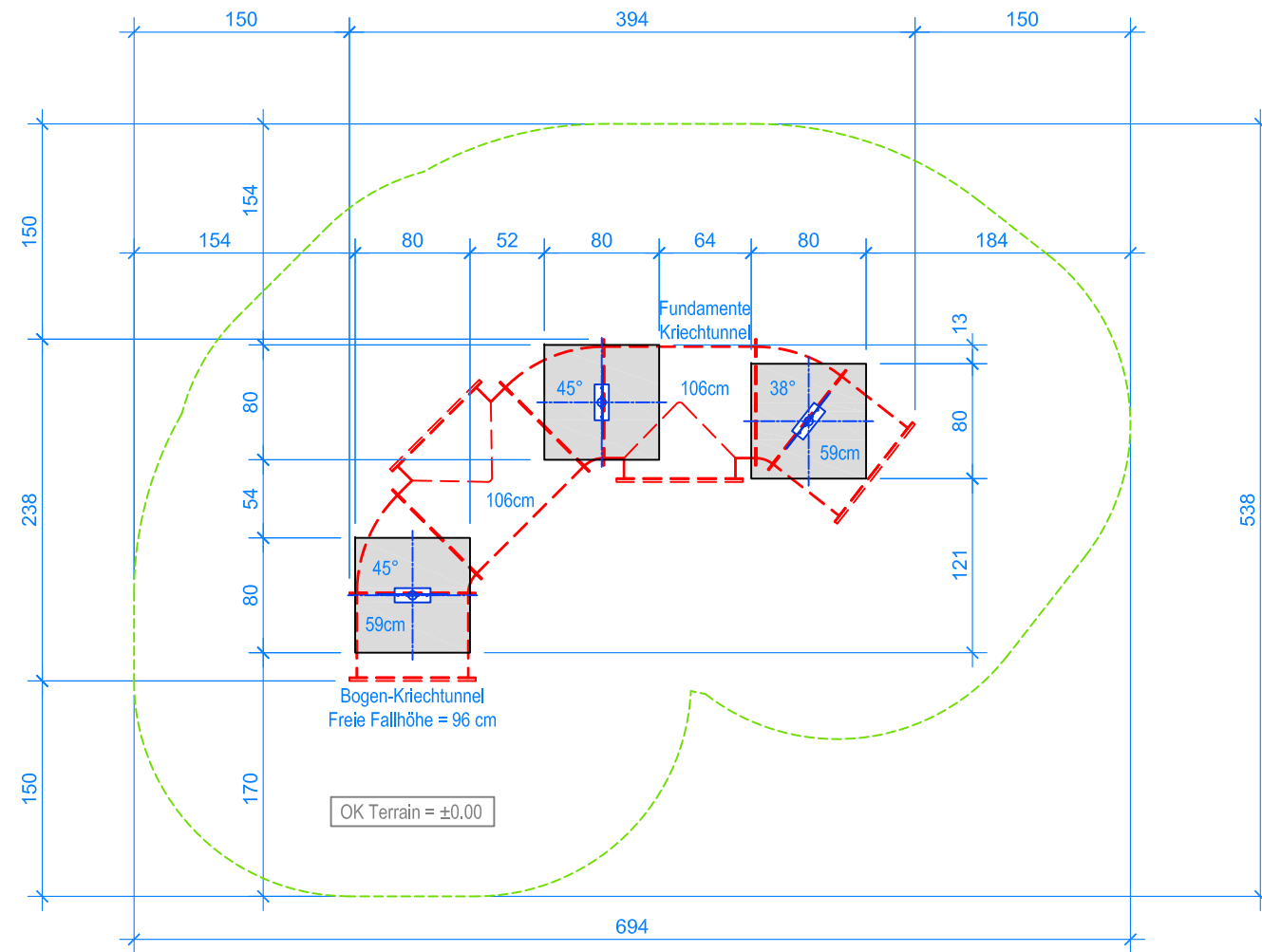
GRUNDRISS 1:50
