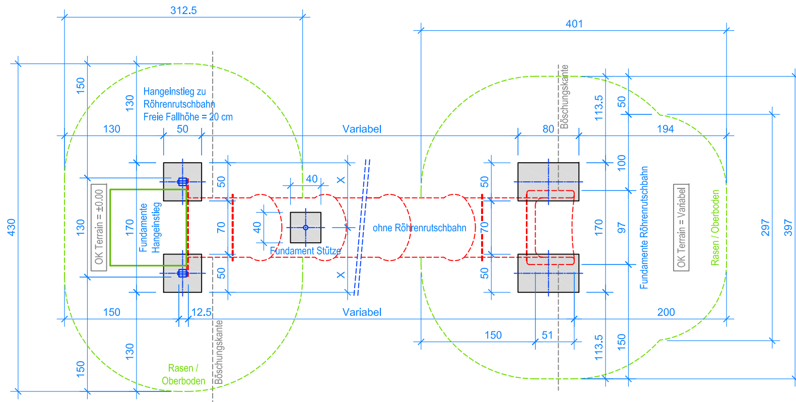
GRUNDRISS 1:50
