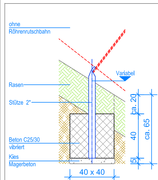
SCHNITT 1:20 FUNDAMENT STÜTZE RÖHRENRUTSCHBAHN
