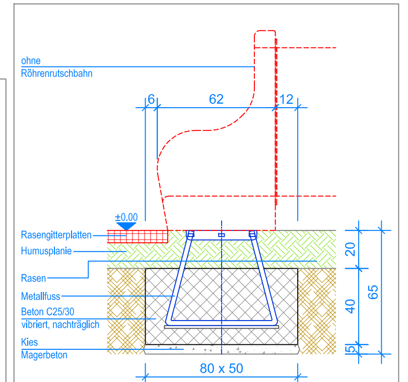
SCHNITT 1:20 FUNDAMENT RÖHRENRUTSCHBAHN
