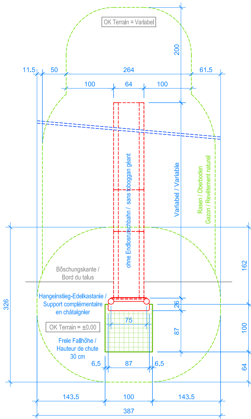
GRUNDRISS / PLAN 1:50
