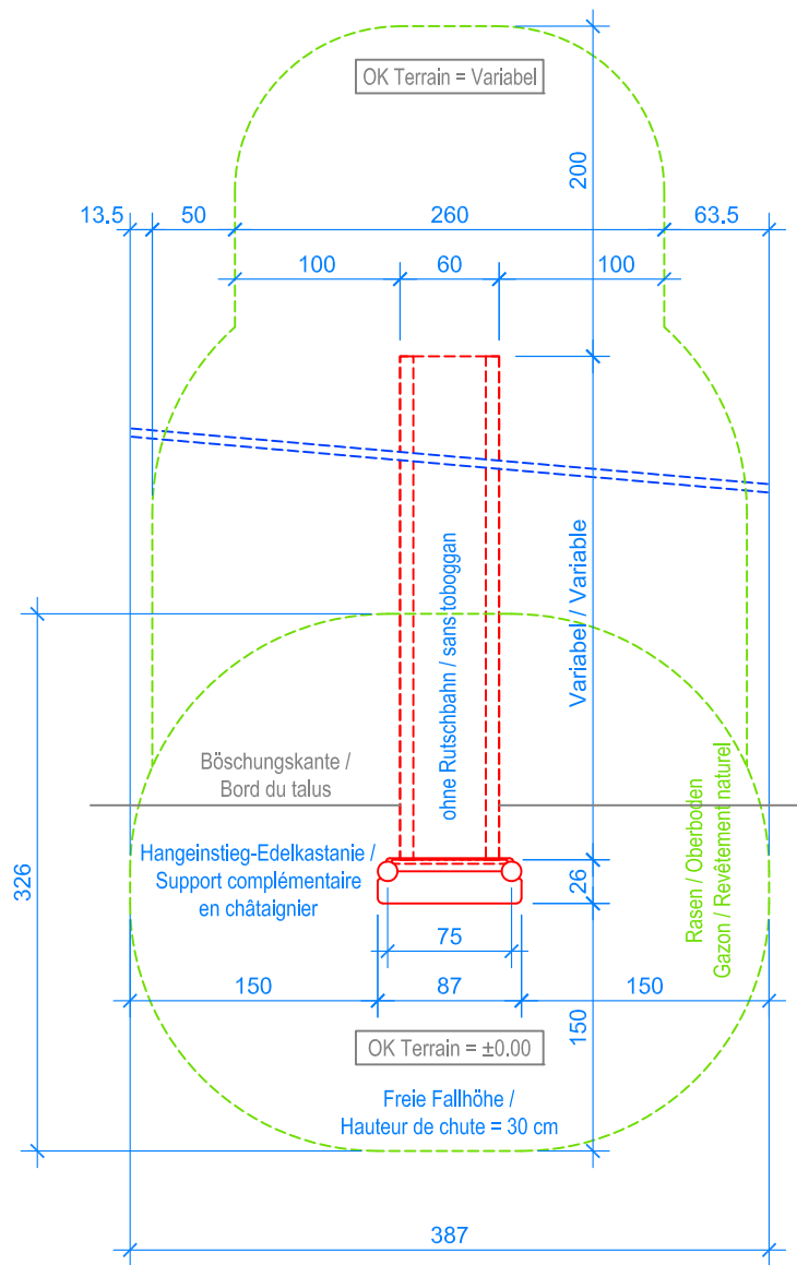
GRUNDRISS / PLAN 1:50
