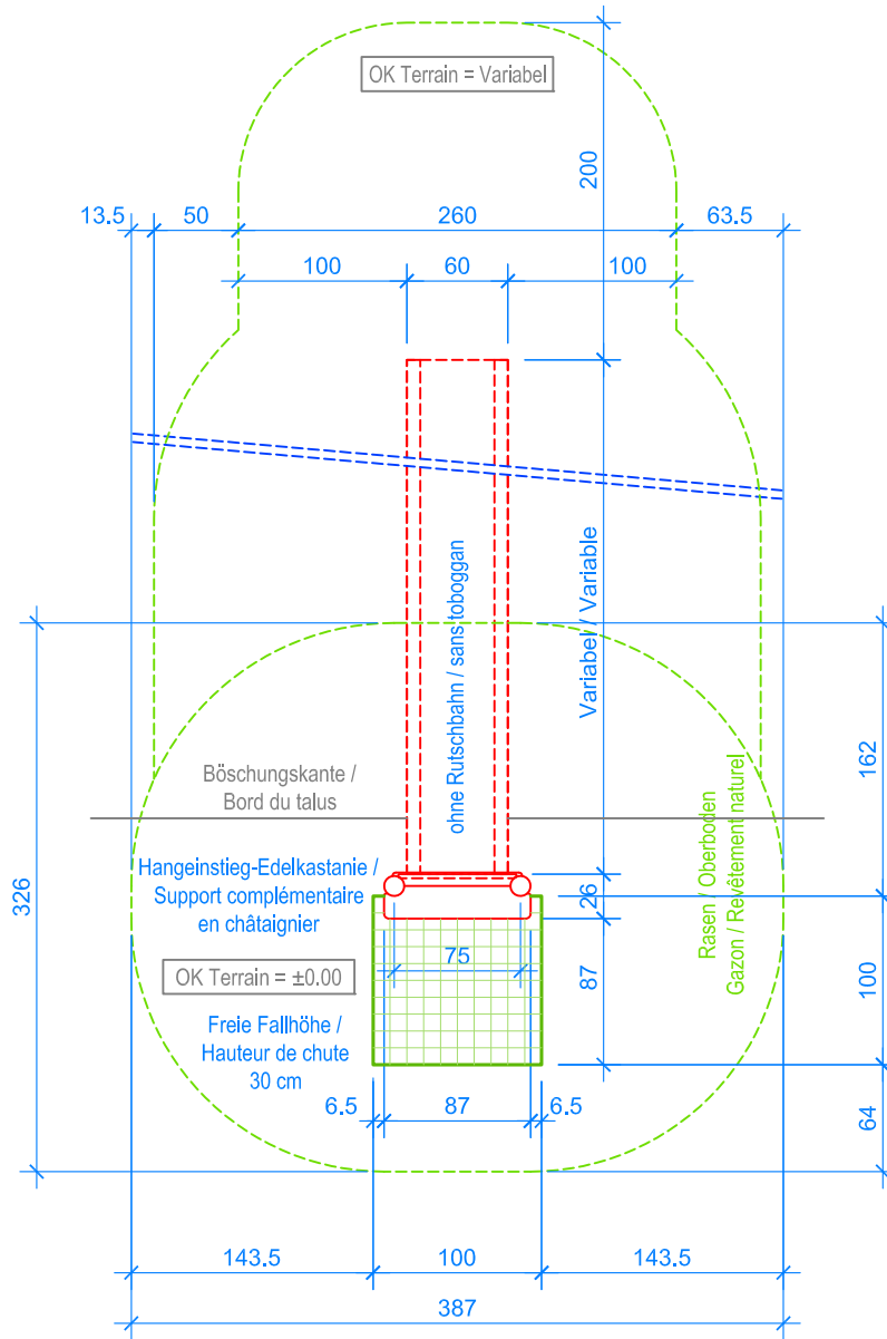
GRUNDRISS / PLAN 1:50
