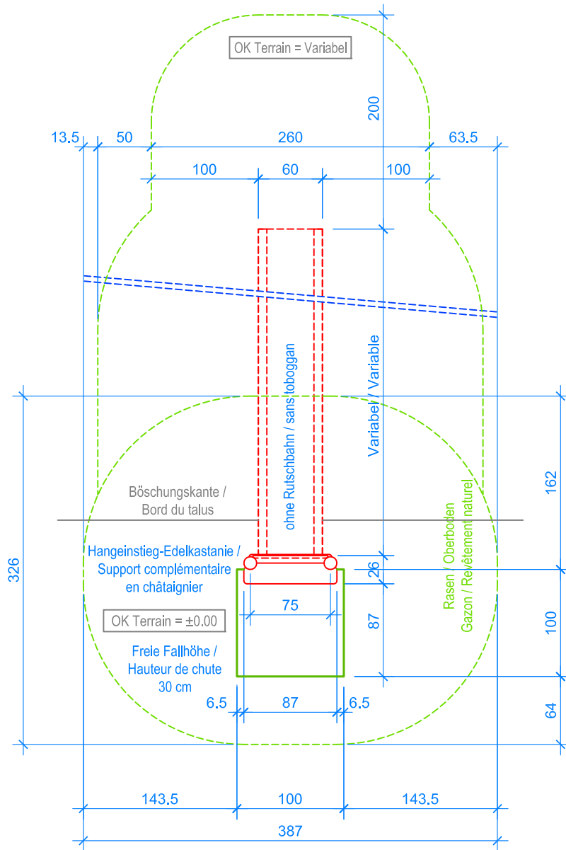
GRUNDRISS / PLAN 1:50
