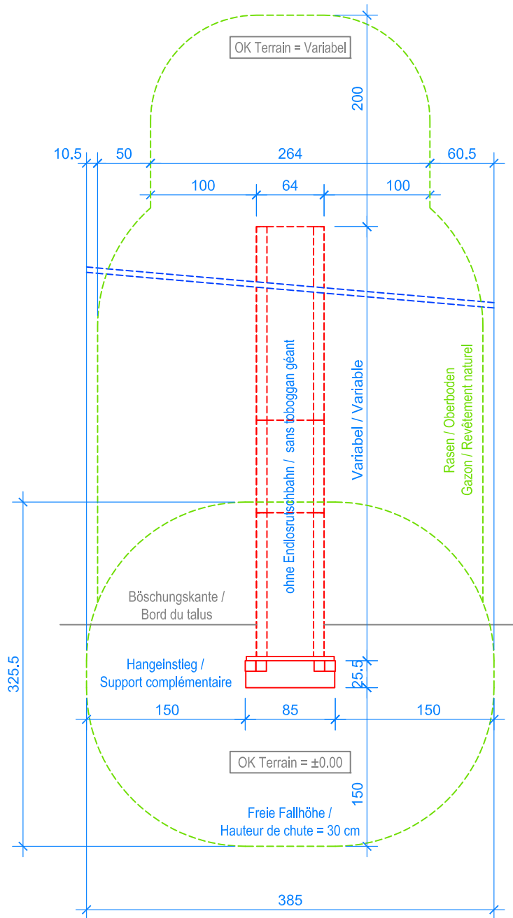
GRUNDRISS / PLAN 1:50
