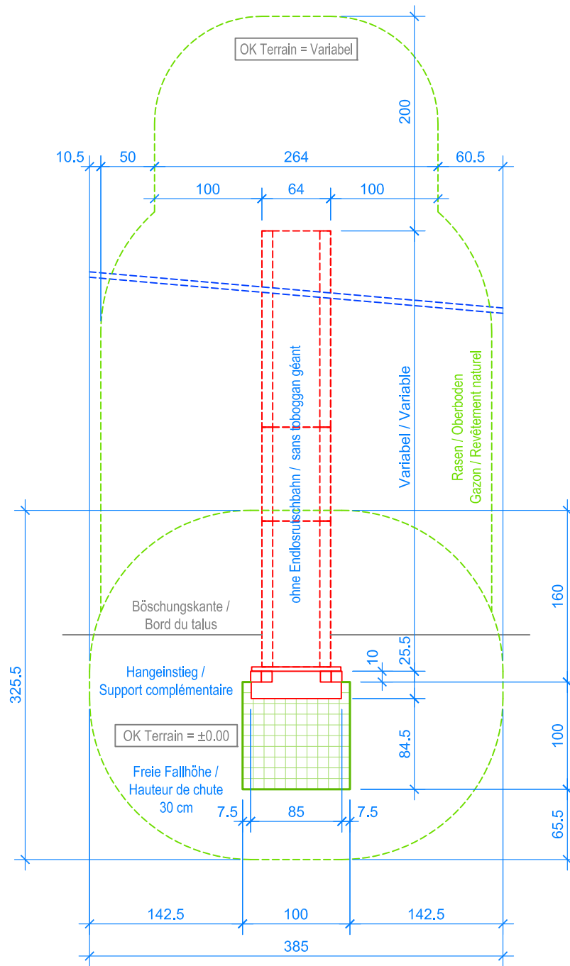
GRUNDRISS / PLAN 1:50
