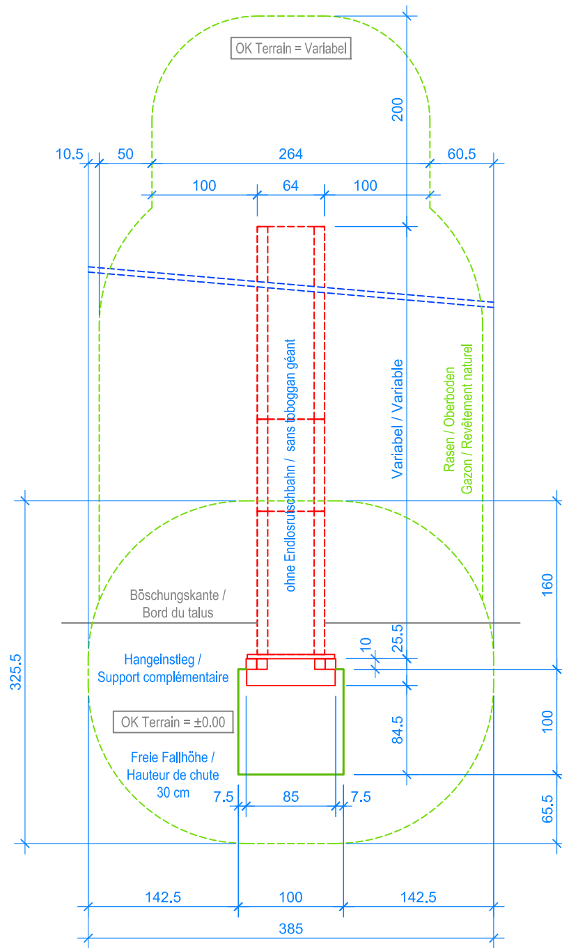
GRUNDRISS / PLAN 1:50
