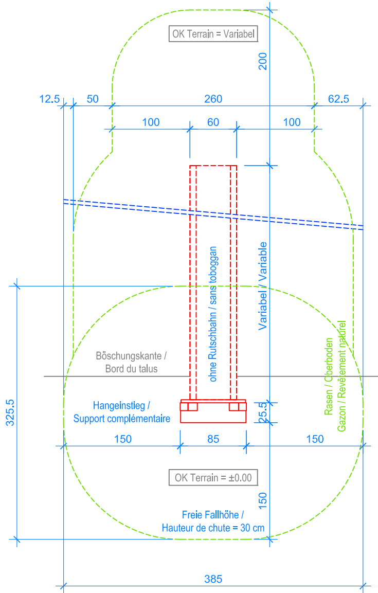
GRUNDRISS / PLAN 1:50
