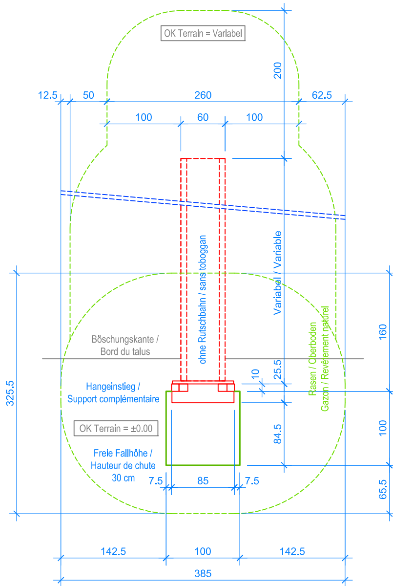
GRUNDRISS / PLAN 1:50
