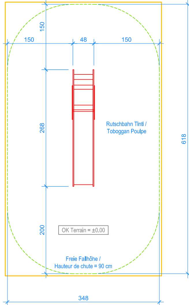
GRUNDRISS / PLAN 1:50
