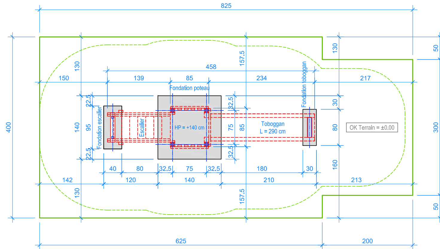
PLAN 1:50
