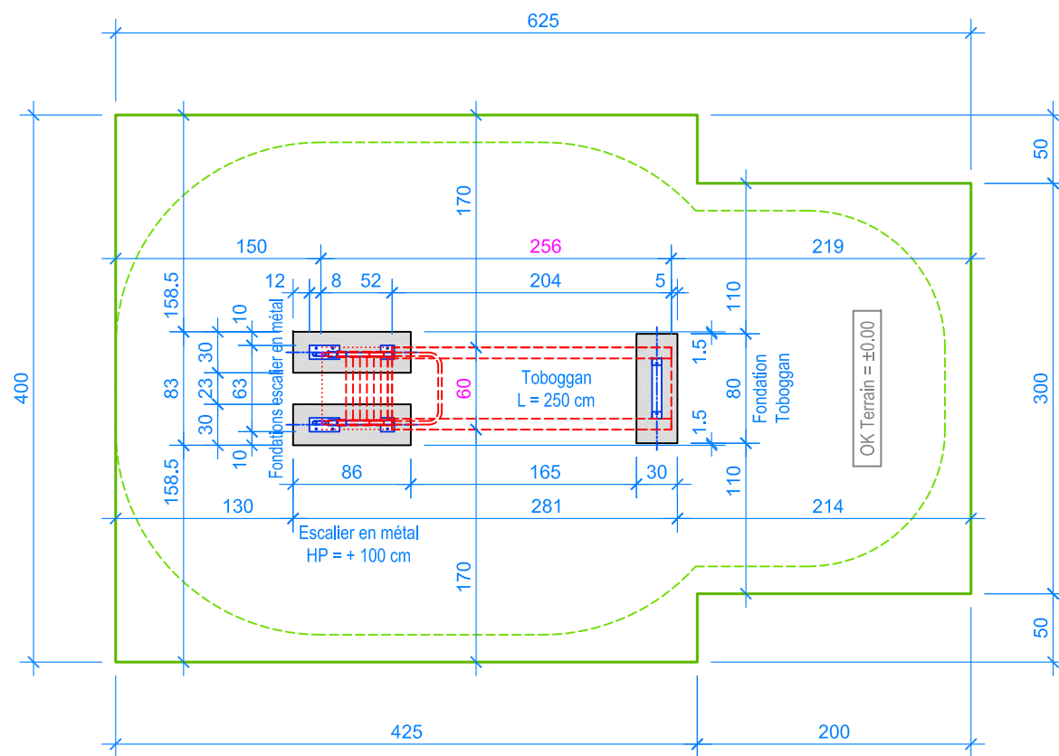
PLAN 1:50
