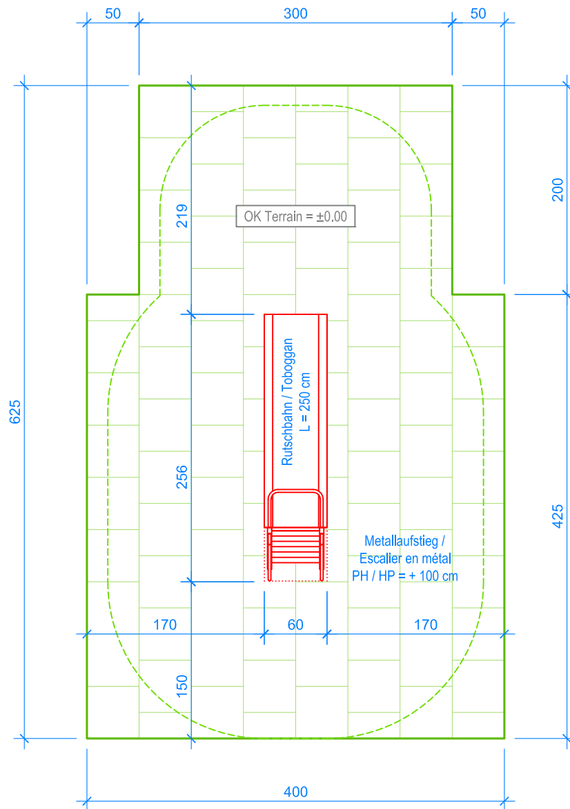
GRUNDRISS / PLAN 1:50
