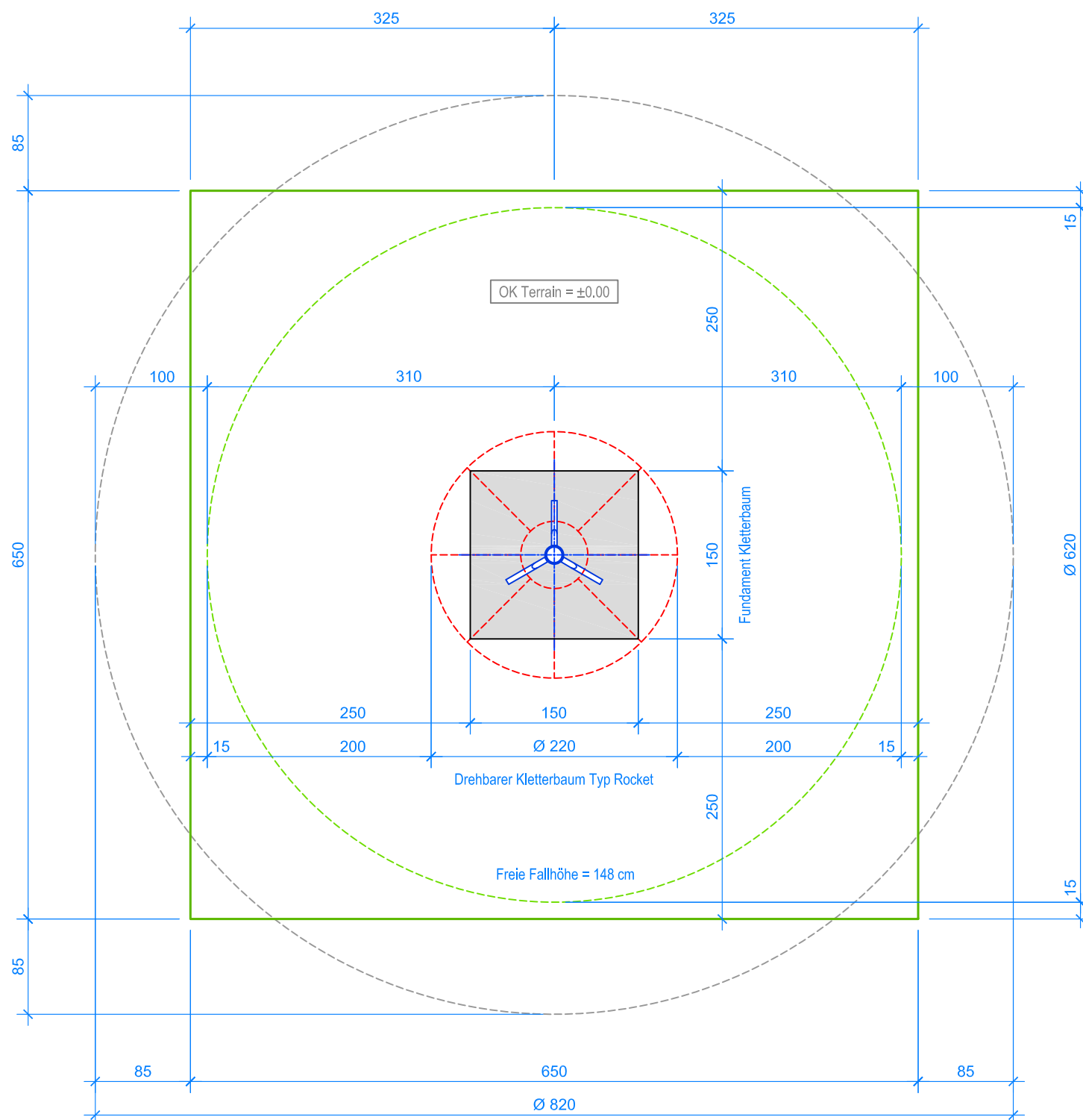
GRUNDRISS 1:50
