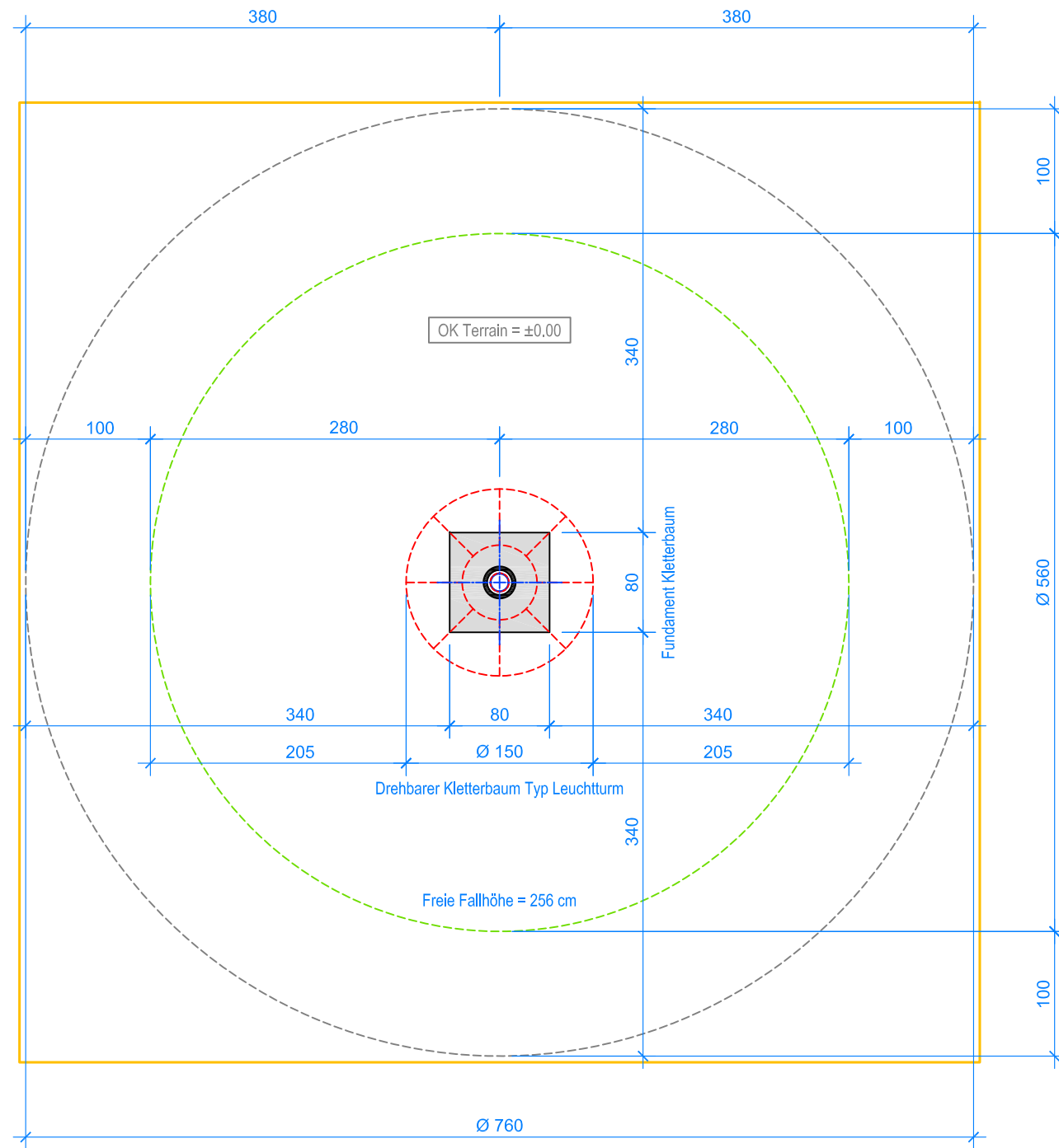
GRUNDRISS 1:50
