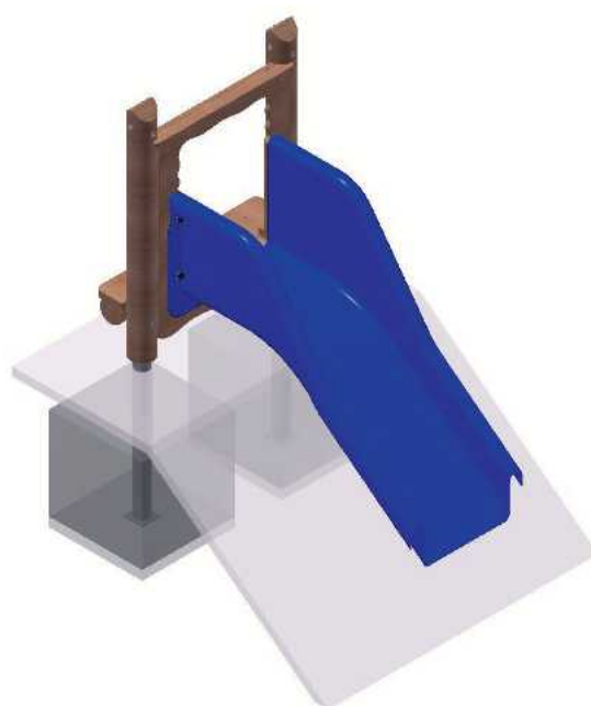
Hangeinstieg aus Edelkastanie zu Endlosrutschbahn Support complémentaire en châtaignier pour départ toboggan géant
